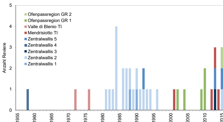
Abb. 9. Jährliche Zahl der Reviere des Brachpiepers Anthus campestris in der Schweiz, differenziert nach den Brutplätzen und den Regionen. – Yearly number of territories of Tawny Pipit Anthus campestris in Switzerland, with indication of the breeding site and the region.
