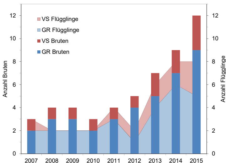
Abb. 4. Jährliche Zahl der Bruten und Flügglinge des Bartgeiers Gypaetus barbatus in der Schweiz seit 2007, differenziert nach den beiden Populationskernen in den Ost- (Graubünden, GR) und Westalpen (Wallis, VS). – Yearly number of broods and fledglings of the Bearded Vulture Gypaetus barbatus in Switzerland since 2007, for the two population nuclei in the Eastern (Grisons, GR) and Western Alps (Valais, VS).
